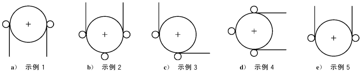
注 1: 分图 a)~d)为符合本条要求的示例。 注 2: 分图 e)为不符合本条要求的示例。
