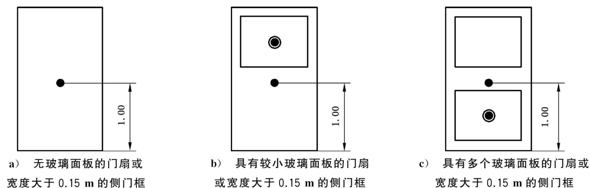
图 11 门和侧门框的摆锤冲击试验——撞击点
