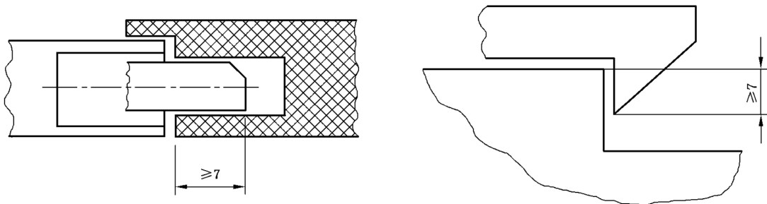
图 12 锁紧部件示例
