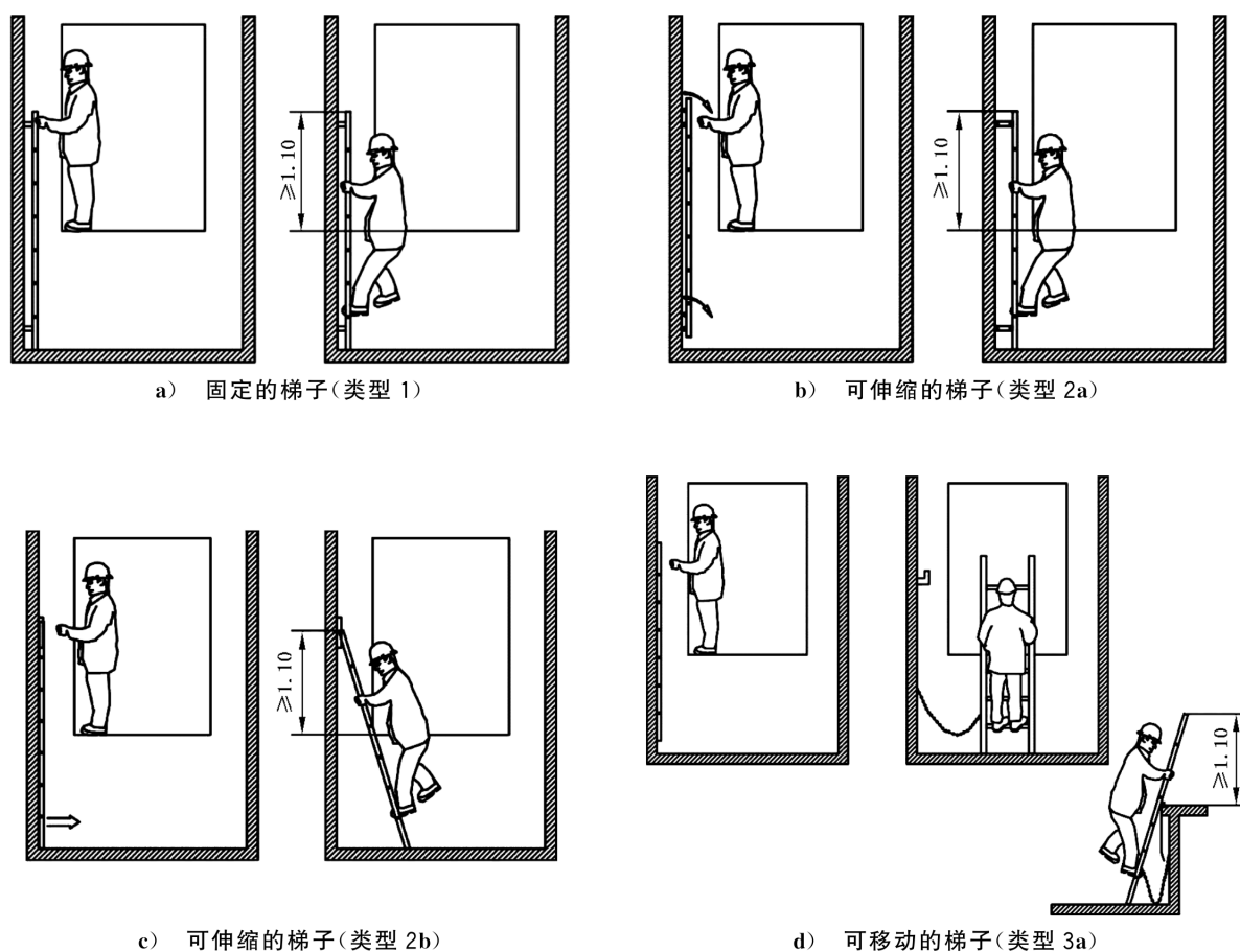
图 F.1 进出底坑梯子的类型
