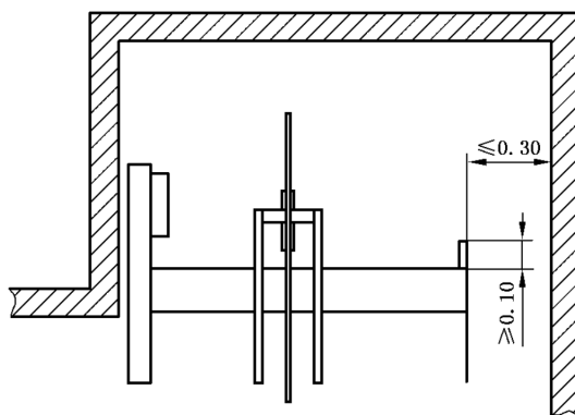
a) 无护栏,但具有最小高度 0.10 m 的踢脚板
