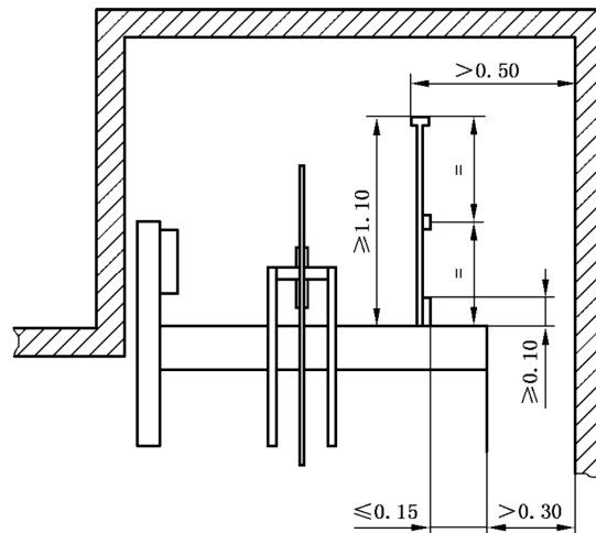
c) 具有最小高度 1.10 m 的护栏和最小高度 0.10 m 的踢脚板
