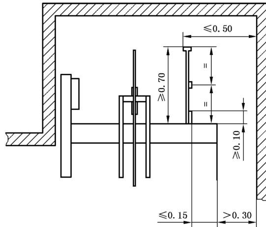
b) 具有最小高度 0.70 m 的护栏和最小高度 0.10 m 的踢脚板
