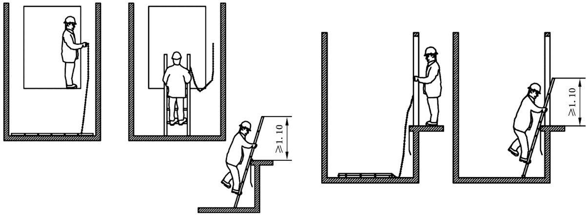
e) 可移动的梯子(类型 3b)
