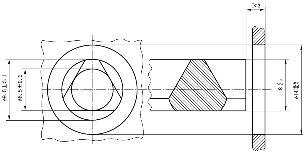
图 13 三角形开锁装置
